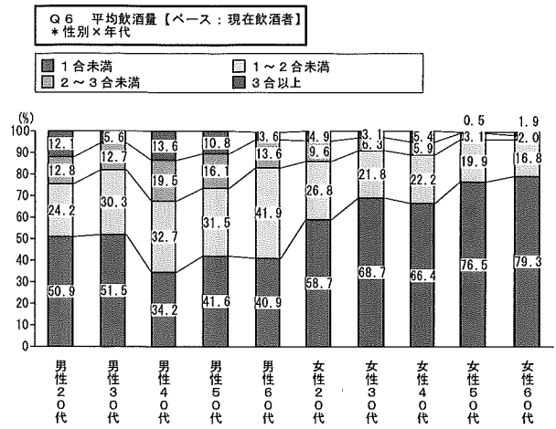
図6 平均飲酒量
