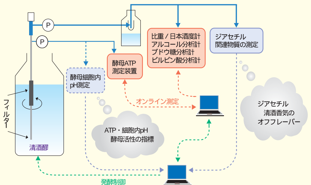
清酒醪のオンライン分析と発酵制御システム
