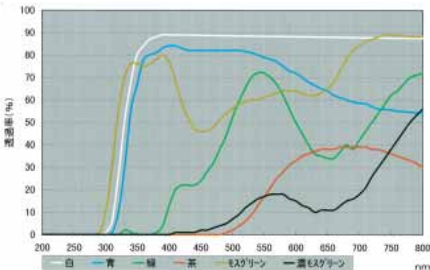
着色びんの透過光スペクトル
